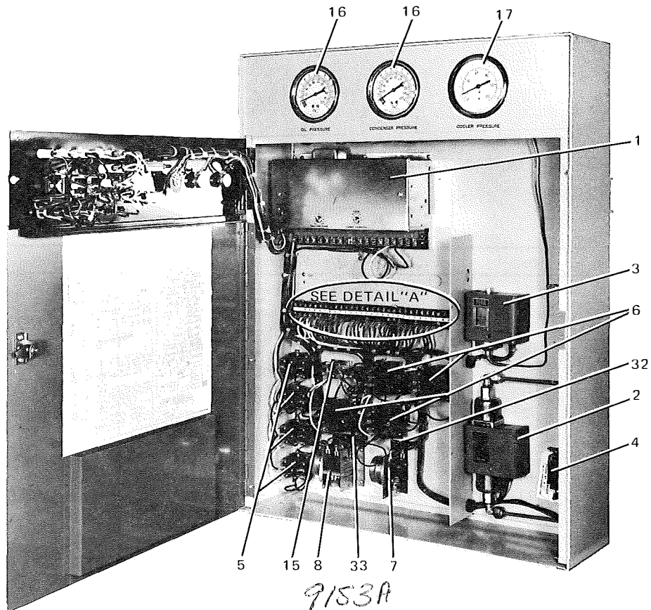
FIG. 24— ELECTRONIC CONTROL CENTER — Panel Part No.'s 367-83019-002, 367-83019-004
