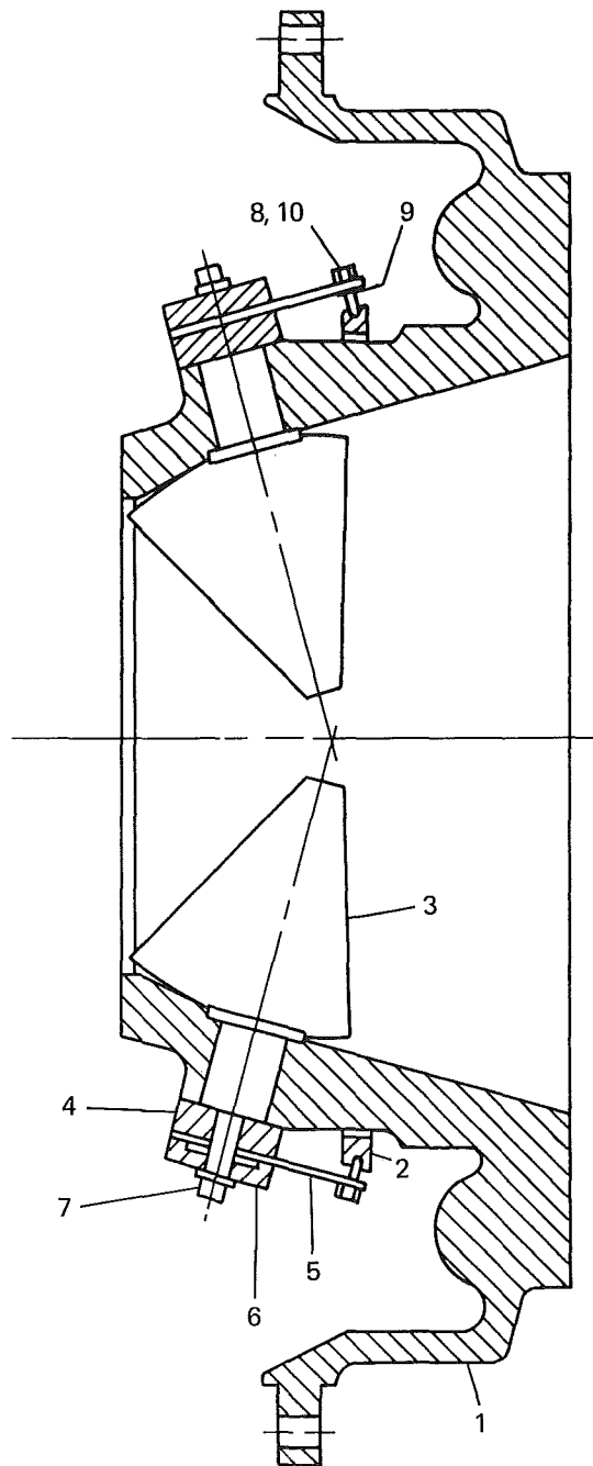
FIG. 7— PRV ASSEMBLY
